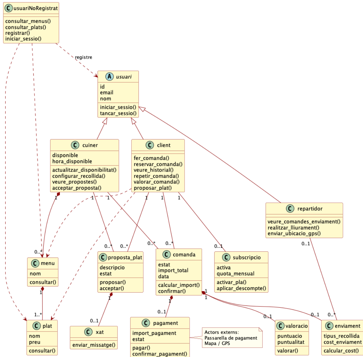
Diagrama de classes – QueMenges (visió general)
